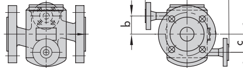
Flanges, DIN 2635
